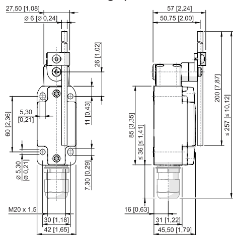
Rod lever 8070/2-4-DD-U60
