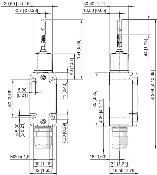
Spring rod 8070/2-2-TK-U60
