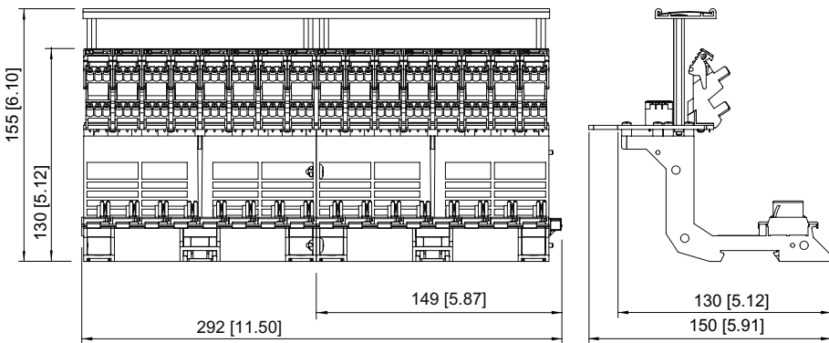
Type 9195/16-...-..., 16 slots
