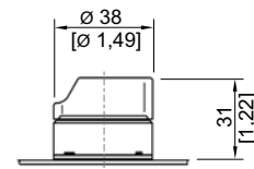
8003/...-726 Poignée rotative
