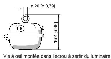
Vis à œil montée dans l'écrou à sertir du luminaire
