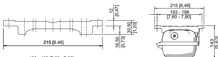
Support rail DIN
