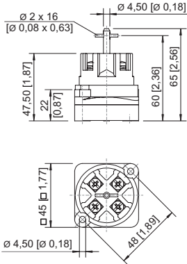
8008/2-0 commutateur de commande 1 ou 2 pôles
