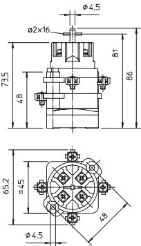
8008/2-6 Sectionneur de charge 3 ou 4 pôles
