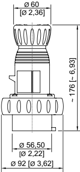
Fiche 5 pôles
