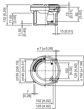
Boîtier taille 2 sans hublot
