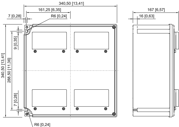
Boîtier 8146/5083 pour coffret batterie 8316/22-24-0100-1
