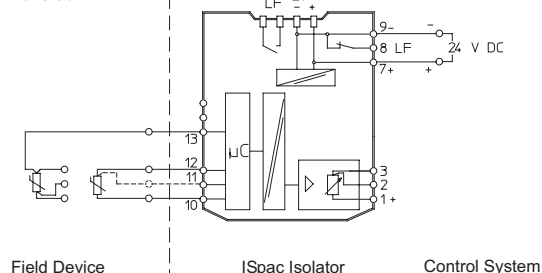
Schéma de raccordement 9180/1.-77-11
