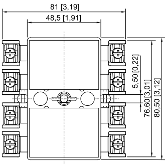
Interrupteur de puissance/moteur série 8006/4, 1 pôle et 2 pôles
