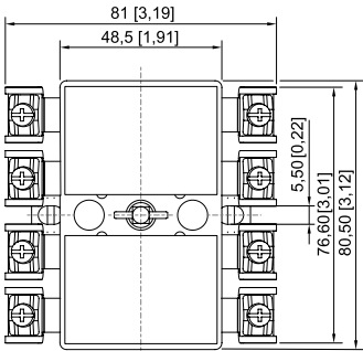
Interrupteur de puissance/moteur série 8006/4, 1 pôle et 2 pôles
