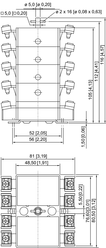
Interrupteur de puissance/moteur série 8006/4, 7 pôles et 8 pôles
