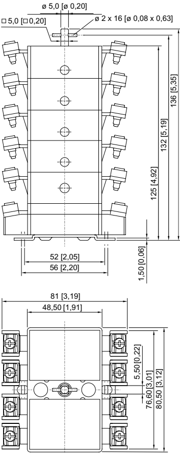
Interrupteur de puissance/moteur série 8006/4, 9 pôles et 10 pôles
