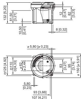
Boîtier taille 1 avec hublot
