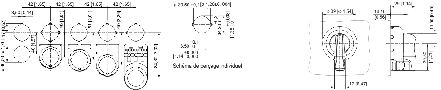
Cotes modulaires de montage avec / sans étiquette de signalisation supplémentaire 8602/3-734 Poignée rotative, verrouillable 1 fois Tête de commande avec actionnement radial
