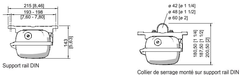
Support rail DIN
