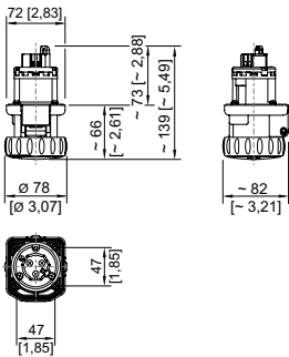
Prise de courant à bride 3 pôles
