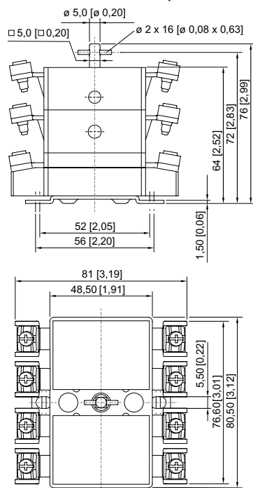
Interrupteur de puissance/moteur série 8006/4, 3 pôles et 4 pôles
