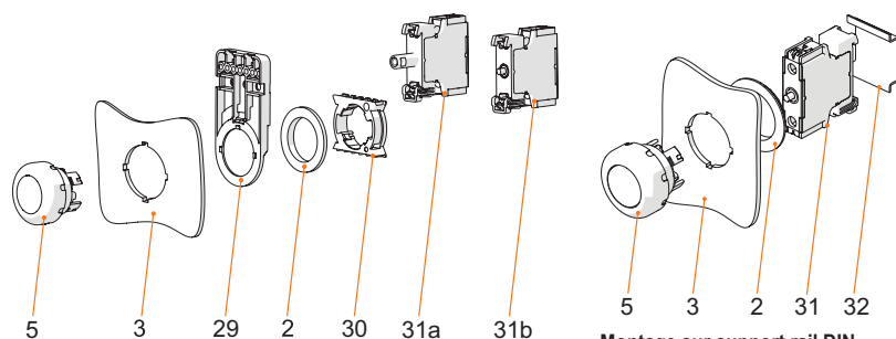
Montage en encastrement frontal avec voyant lumineux série 8010/6 et élément de contact série 8082/3
