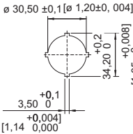
Schéma de perçage individuel
