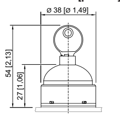
8003/...-008 Commutateur à clé
