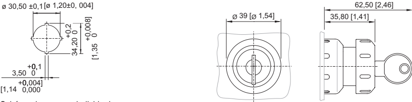
Schéma de perçage individuel
