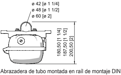
Abrazadera de tubo montada en rail de montaje DIN
