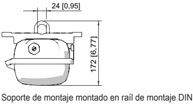
Soporte de montaje montado en rail de montaje DIN
