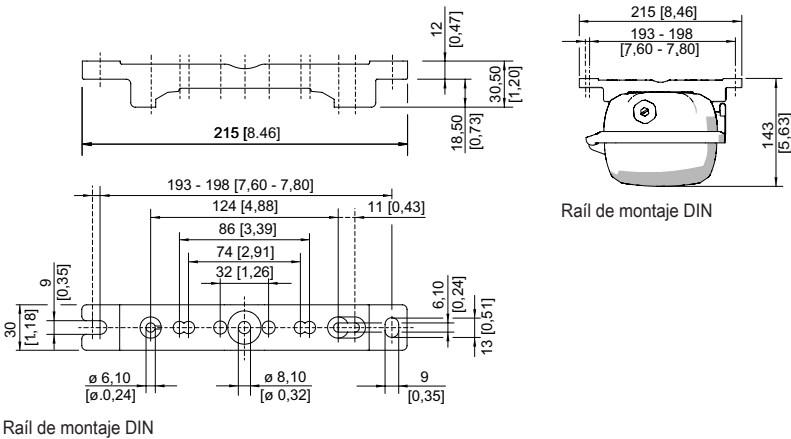
Rail de montaje DIN
