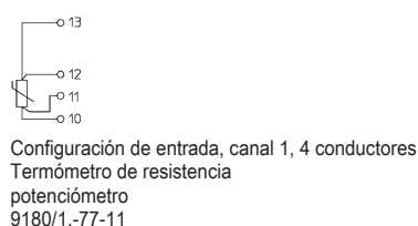
Diagrama de conexión 9180/1.-77-11
