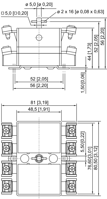
Interrupor de carga y motor, serie 8006/4, de 1 y 2 polos
