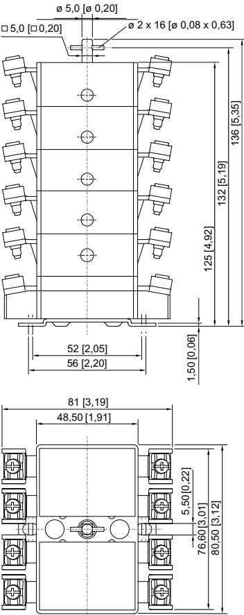
Interrupor de carga y motor, serie 8006/4, de 9 y 10 polos
