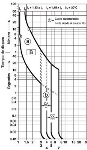
Caracterstica de disparo B
