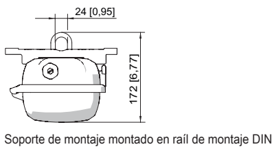
Soporte de montaje montado en raíl de montaje DIN
