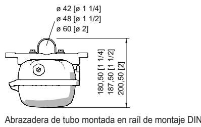
Abrazadera de tubo montada en raíl de montaje DIN
