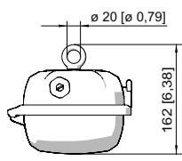
Tornillo de cáncamo montado en tuerca autoinsertable de la luminaria
