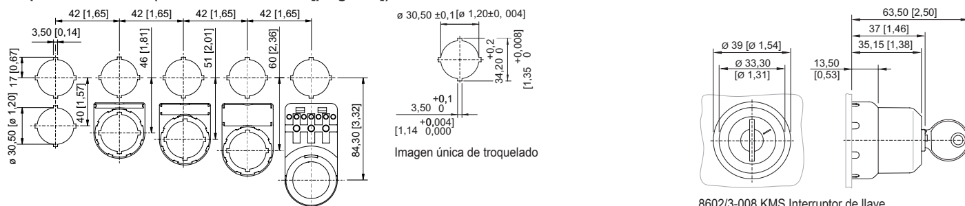
8602/3-008 KMS Interruptor de llave Pieza de accionamiento con accionamiento axial
