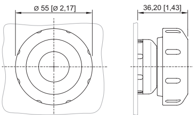
8602/3-014 Pulsador seta rojo/negro 8602/3-703 Pulsador seta negro/negro Actuador con accionamiento axial
