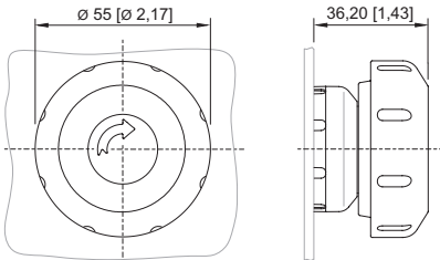
8602/3-015 Pulsador seta enclavable rojo/amarillo Actuador con accionamiento axial
