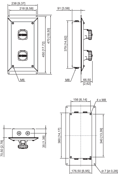
8150/5-V88 con 8572/15, 16 A
