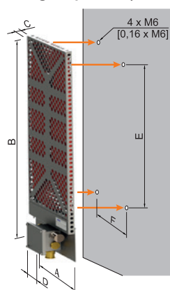
4 x fori di montaggio Ø 6 mm sul retro del riscaldamento
